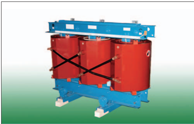
Сухий трансформатор з епоксидною ізоляцією типу GEAFOL виробництва компанії Siemens
